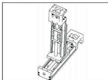
LA20-BS ... XY-T
