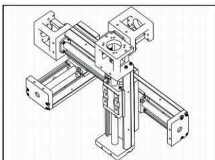
LA20-BS ... XYZ-X
